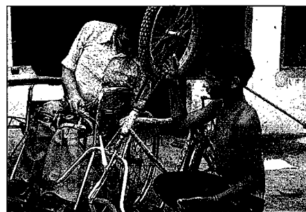
Leopoldo Leyva, un fabricante de sillas de ruedas de PROJIMO, solda la bicicleta de un niño.
